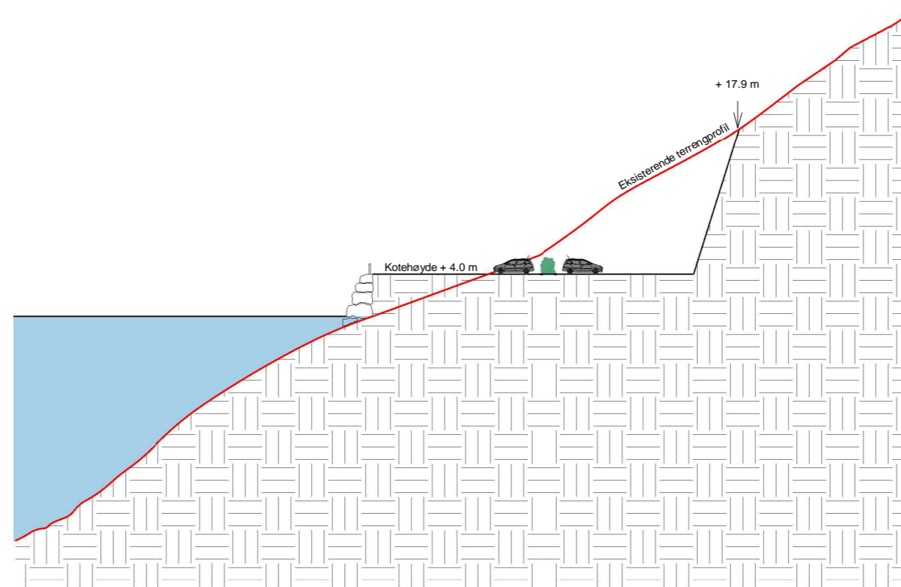
2 Snitt 2 1 : 500
