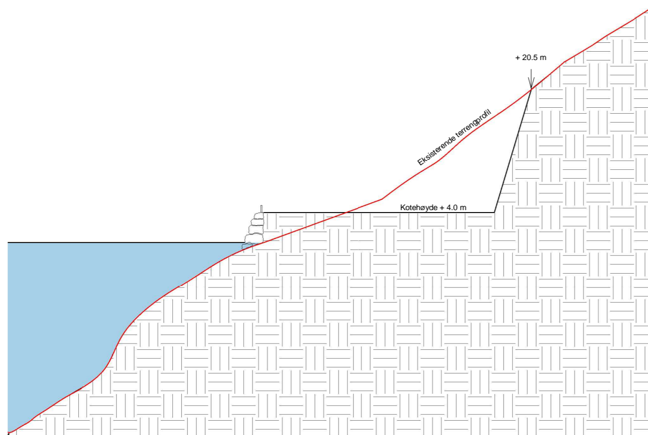
3 Snitt 3 1 : 500
